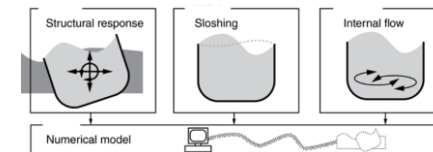
Prinsippskisse påføring; lukket merd. Illustrasjon AkvaDesign AS
