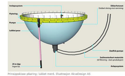
Prinsippskisse påføring; lukket merd. Illustrasjon AkvaDesign AS
